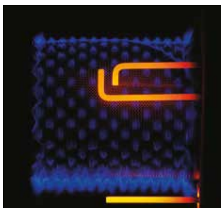
Bruciatore Matrix cilindrico con modulazione fino a 1:7
